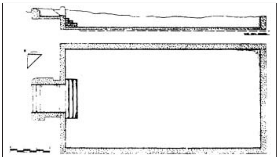
Planta elaborada per J.M. Solías de l'estructura de la vil·la romana que es troba al municipi
